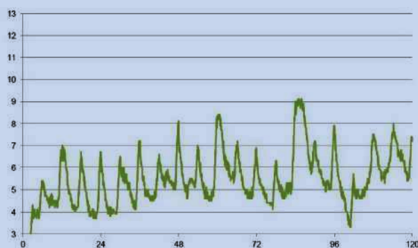
Η ΘΕΡΜΟΚΡΑΣΙΑ ΤΩΝ ΠΙΤΩΝ ΣΕ ΨΥΚΤΙΚΟ ΘΑΛΑΜΟ ΜΕ ΚΟΥΡΤΙΝΕΣ PVC
